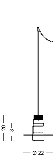
1403.3L Sospensione / Hanging lamp vetro/glass Ø22 cm - cavo/cable 200 cm 3x LED 10W - 3000 K - 900 lm - 230V CE IP20 1m
