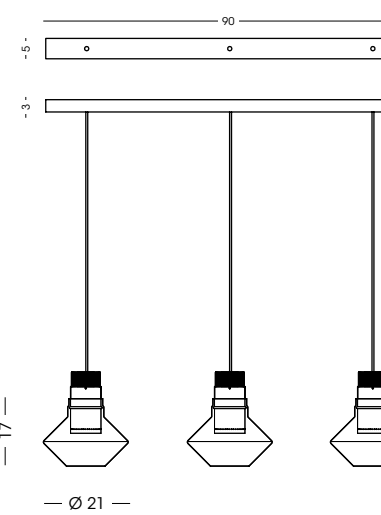
1447.90.3L Binario a soffitto / Ceiling track vetro/glass Ø21 cm - cavo/cable 200 cm 3x LED 10W - 3000 K - 900 lm - 230V CE IP20 1m
