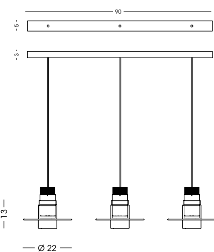
1407.90.3L Binario a soffitto / Ceiling track vetro/glass Ø22 cm - cavo/cable 200 cm 3x LED 10W - 3000 K - 900 lm - 230V CE IP20 1m
