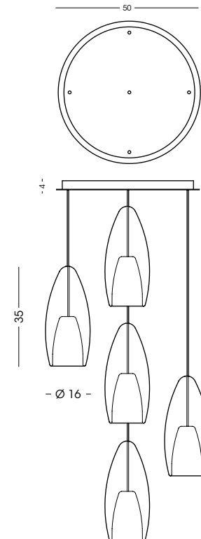
GIG1399.50.5L Plafoniera / Ceiling lamp vetro/glass Ø16 cm - cavo/cable 200 cm 5 E27 x 105W 220-240V CE IP20 1m
