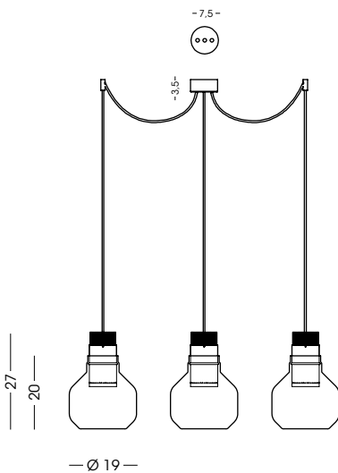
1413.3L Sospensione / Hanging lamp vetro/glass Ø19 cm - cavo/cable 200 cm 3x LED 10W - 3000 K - 900 lm - 230V CE IP20 1m
