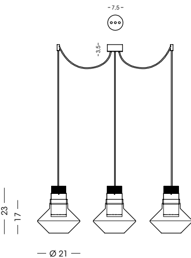
1443.3L Sospensione / Hanging lamp vetro/glass Ø21 cm - cavo/cable 200 cm 3x LED 10W - 3000 K - 900 lm - 230V CE IP20 1m
