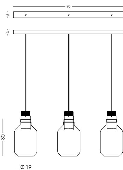
1427.90.3L Binario a soffitto / Ceiling track vetro/glass Ø19 cm - cavo/cable 200 cm 3x LED 10W - 3000 K - 900 lm - 230V CE IP20 1m
