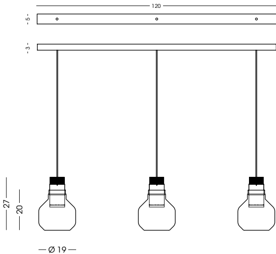
1417.120.3L Binario a soffitto / Ceiling track vetro/glass Ø19 cm - cavo/cable 200 cm 3x LED 10W - 3000 K - 900 lm - 230V CE IP20 1m
