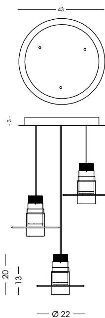
1407.120.3L Binario a soffitto / Ceiling track vetro/glass Ø22 cm - cavo/cable 200 cm 3x LED 10W - 3000 K - 900 lm - 230V CE IP20 1m
