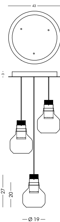
1417.120.3L Binario a soffitto / Ceiling track vetro/glass Ø19 cm - cavo/cable 200 cm 3x LED 10W - 3000 K - 900 lm - 230V CE IP20 1m
