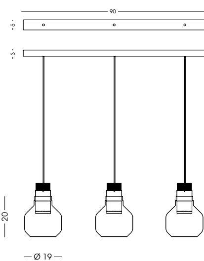
1417.90.3L Binario a soffitto / Ceiling track vetro/glass Ø19 cm - cavo/cable 200 cm 3x LED 10W - 3000 K - 900 lm - 230V CE IP20 1m
